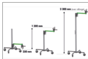
Bohrhöhe von 250 bis 1 300 mm
