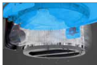
HEPA 13-Patronenfilter mit zwei unabhängigen Filterkammern
