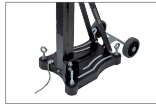
Embase mixte, à cheviller / dépression ; aiguille de centrage
