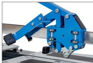
Tête de coupe montée sur 11 roulements à billes
