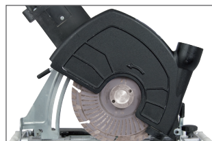
Réglage de l'inclinaison de coupe par palier, jusqu'à 45° sans outil complémentaire
