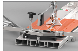
Châssis et support de rail en aluminium
