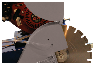
Système d'ouverture du carter = changement de disque facilité
