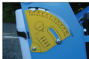
Indicateur de la profondeur de coupe en fonction du diamètre du disque
