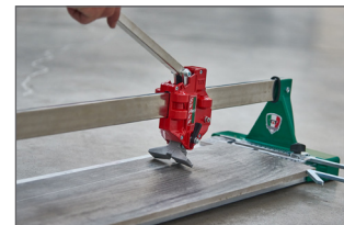
Séparateur de coupe : une simple pression du levier suffit
