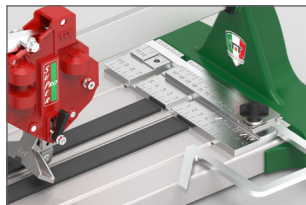
Support de carrelage en aluminium avec une échelle millimétrique très visible
