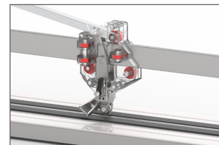
Chariot avec 9 roulements à billes, dont 4 réglables : coulissage parfait et grande précision
