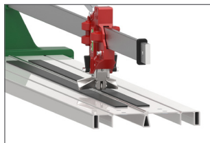
Châssis robuste en aluminium : rigidité et légèreté à la fois
