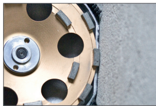
Avant du carter amovible pour le ponçage au ras du mur
