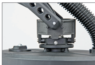
Système anti-vibratoire articulé monté sur ressorts = compense les irrégularités
