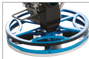
Pales arrivant au ras du carter pour un travail au ras des murs.
