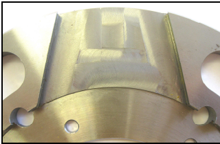
2 Sicherungsschrauben M6x6
